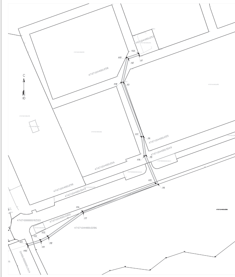
Схема границ земель, предполагаемых к использованию под размещение объекта: «2КЛ-10 кВ от РТП-3351 до проектируемой 2БКТП-10/0,4 кВ в г. Кудрово Всеволожского района ЛО» Месторасположение: Ленинградская область, Всеволожский район, г. Кудрово» в границах земельных участков с кадастровыми номерами 47:07:1044001:5049, 47:07:0000000:91533, 47:07:1044001:11810, 47:07:1044001:2286. Площадь, предполагаемая к использованию 895 м 2 .
